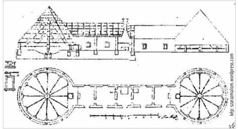
Kiss József: Bácskai szárazmalom tervrajza
